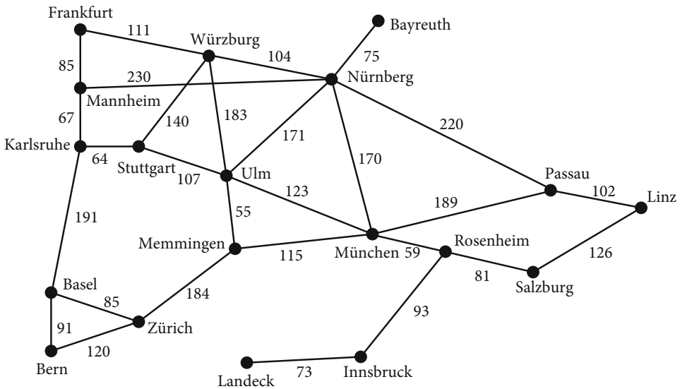
Abb. 6.5 Der Süddeutschlandgraph als Beispiel für eine Suchaufgabe mit Kostenfunktion
