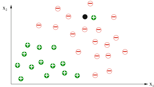
Abb. 8.15 Die Nearest Neighbour-Methode weist hier dem neuen schwarz markierten Punkt die falsche (positive) Klasse zu, denn der nächste Nachbar ist sehr wahrscheinlich falsch klassifiziert
