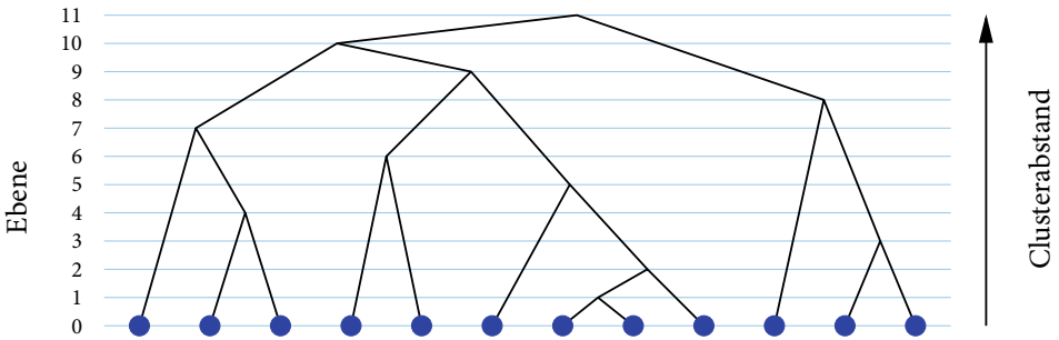
Abb. 8.34 Beim hierarchischen Clustering werden in jedem Schritt die zwei Cluster mit dem kleinsten Abstand vereinigt
