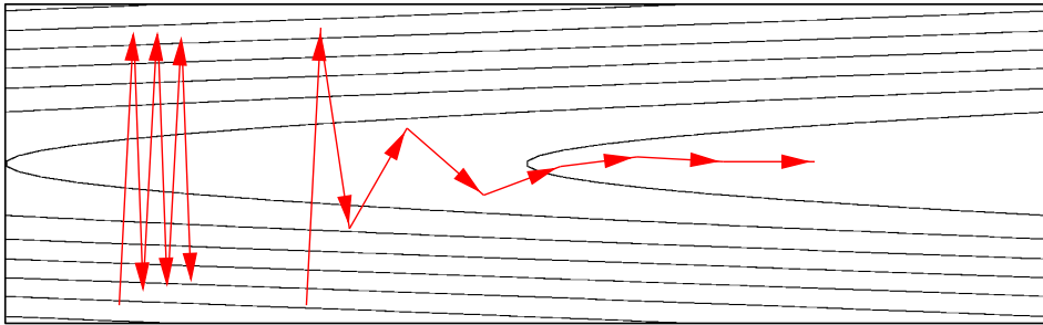
Abb. 9.24 Durch die Verwendung des Impulsterms werden abrupte Richtungsänderungen geglättet. Eine Iteration ohne Impuls-Term ( links ) im Vergleich zur Iteration mit Impuls-Term ( rechts )
