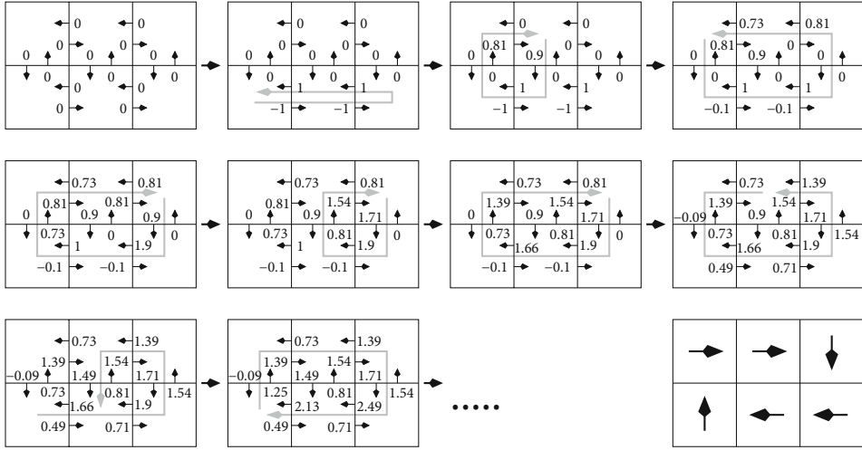
Abb. 10.12 Q-Lernen angewandt auf das Beispiel mit n_x = 3, n_y = 2 . Die grauen Pfeile markieren die im jeweiligen Bild ausgeführten Aktionen. Die aktualisierten Q -Werte sind angegeben. Im letzten Bild ist die aktuelle und zugleich optimale Strategie dargestellt
