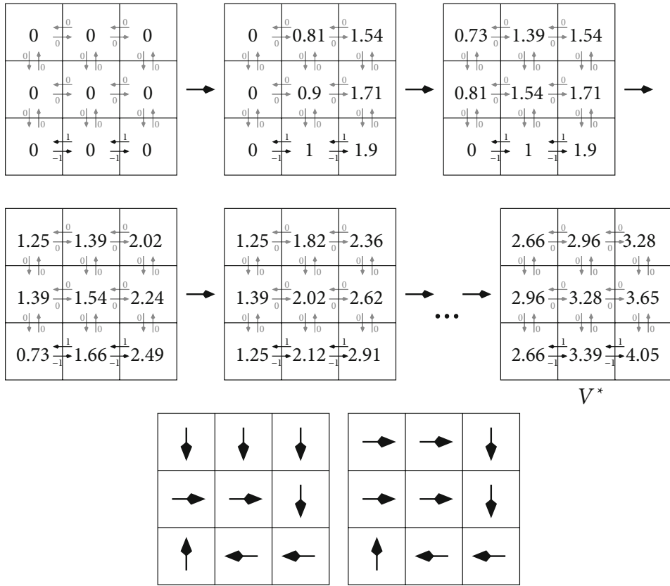
Abb. 10.8 Wert-Iteration am Beispiel mit 3 \times 3 Zuständen. Die letzten beiden Bilder zeigen zwei optimale Strategien. Die Zahlen neben den Pfeilen geben die direkte Belohnung r(s, a) der jeweiligen Aktion an
