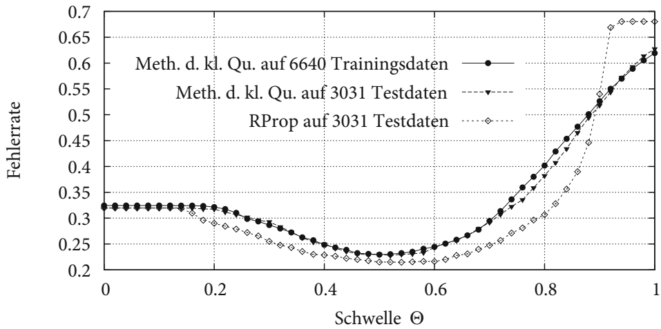
Abb. 9.14 Fehler der Methode der kleinsten Quadrate auf den Trainings- und Testdaten
