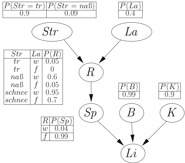
Abb. 11.1 Bayes-Netz für die Fahrradlichtanlage. Die CPT für Li ist in der Aufgabenstellung angegeben
