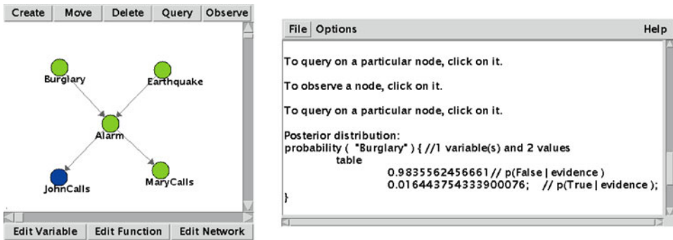
Abb. 7.13 Die Benutzeroberfläche von JavaBayes: Links der graphische Editor und rechts die Konsole, auf der die Antworten ausgegeben werden
