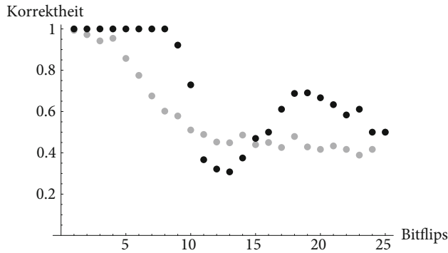
Abb. 8.17 Relative Korrektheit der Nearest Neighbour-Klassifikation in Abhängigkeit von der Zahl invertierter Bits. Die Struktur der Kurve mit dem Minimum bei 13 und Maximum bei 19 hängt mit der speziellen Struktur der Trainingsmuster zusammen. Zum Vergleich sind in grau die Werte des Perzeptrons aus Beispiel 8.3 eingezeichnet
