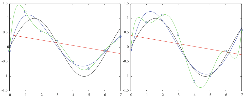
Abb. 8.27 Auf zwei unterschiedlichen Datenmengen wurden Polynome der Grade 1, 4 und 7 approximiert. Man erkennt gut den Bias-Variance-Tradeoff
