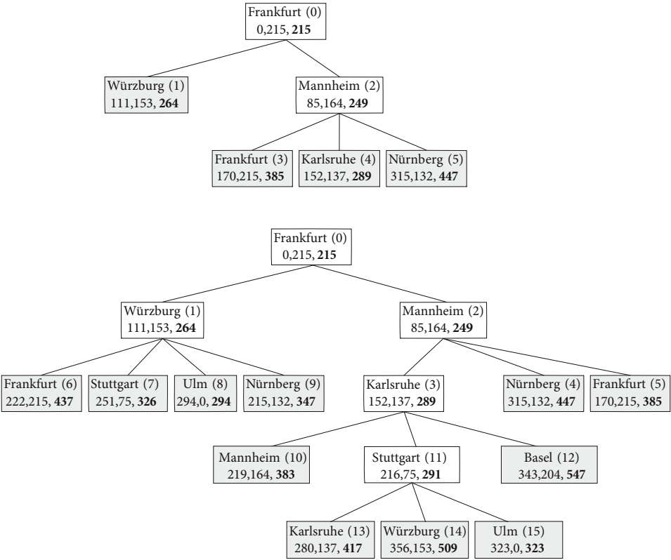
Abb. 6.16 Zwei Momentaufnahmen des Suchbaums der A*-Suche für eine optimale Route von Frankfurt nach Ulm. Unter dem Namen der Stadt s ist jeweils g(s) , h(s) , f(s) angegeben. Nummern in Klammer neben einem Städtenamen geben die Reihenfolge der Erzeugung des Knotens durch die Funktion „Nachfolger“ an
