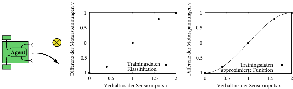
Abb. 8.18 Der lernende Agent, der dem Licht ausweichen soll ( links ), dargestellt als Classifier ( Mitte ) und als Approximation ( rechts )
