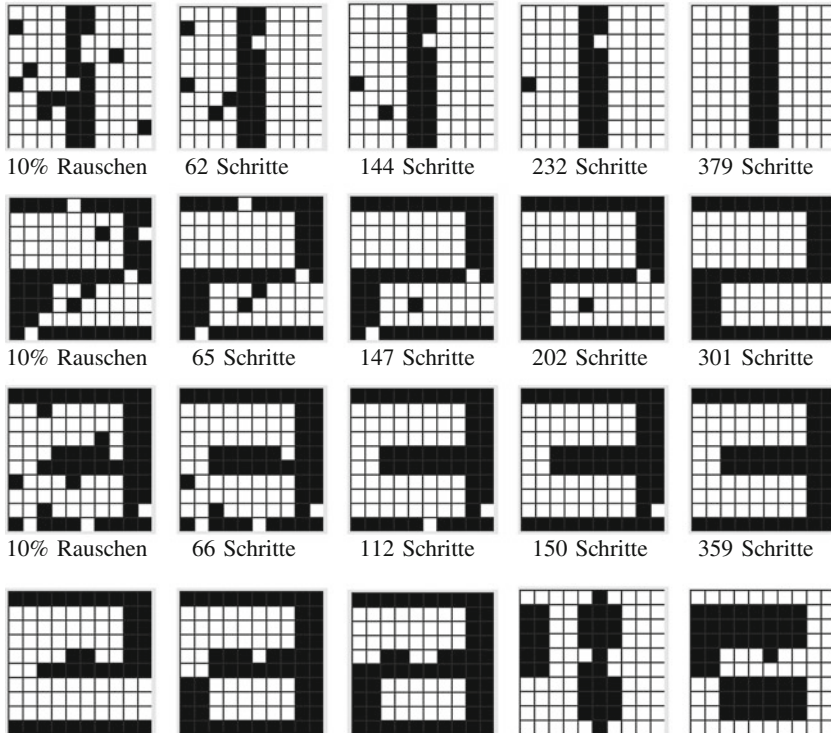
Einige stabile Zustände des Netzes, die nicht gelernt wurden.
