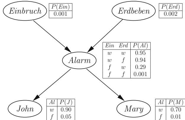
Abb. 7.11 Bayes-Netz für das Alarm-Beispiel mit den zugehörigen CPTs
