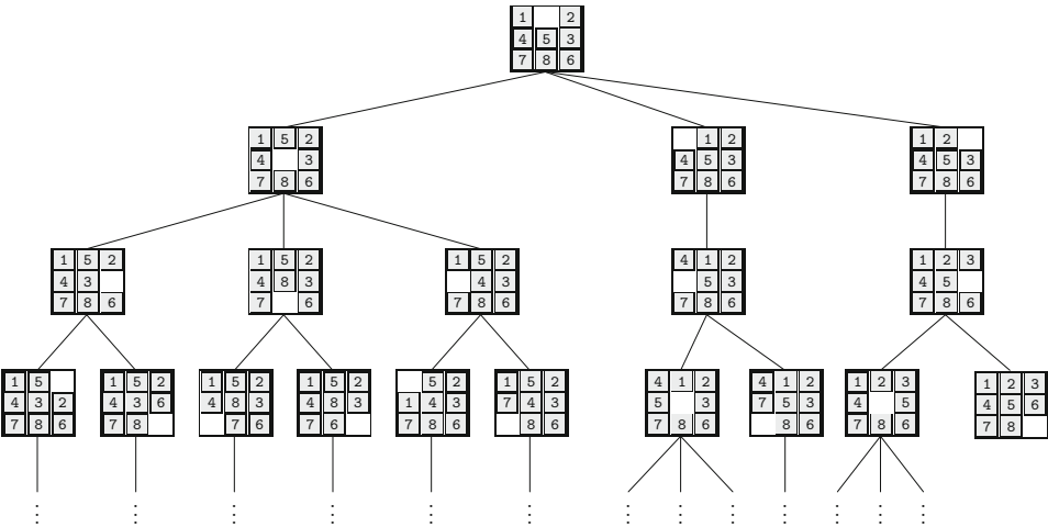
Abb. 6.4 Suchbaum beim 8-Puzzle ohne Zyklen der Länge 2
