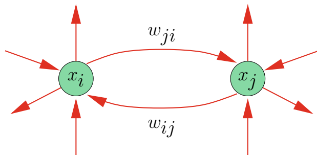
Abb. 9.5 Rekurrente Verbindung von zwei der Neuronen aus einem Hopfield-Netz
