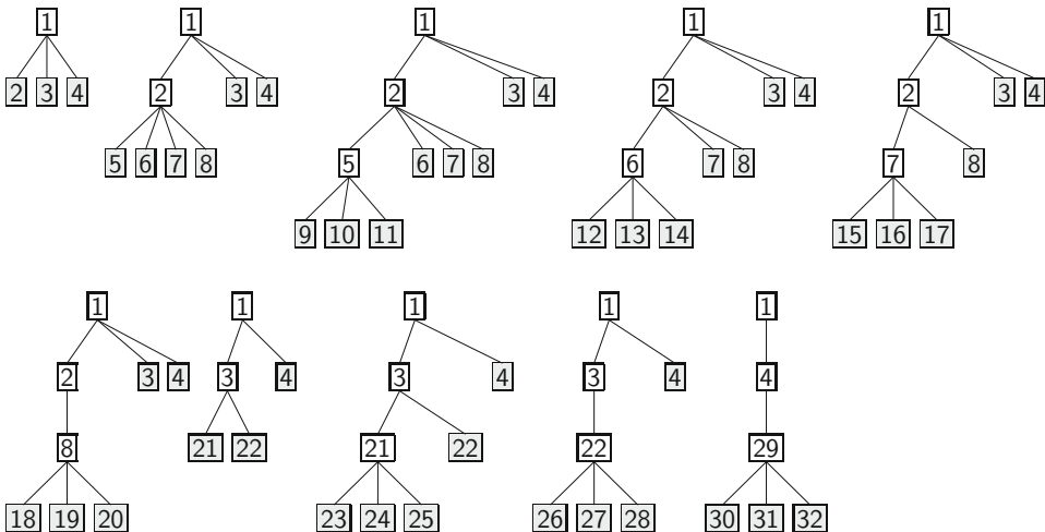
Abb. 6.9 Ablauf der Tiefensuche. Alle Knoten auf Tiefe drei sind erfolglos und führen zum Backtracking. Die Knoten sind nummeriert nach der Reihenfolge ihrer Erzeugung
