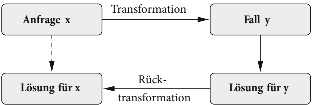
Abb. 8.21 Ist ein zum Fall x ähnlicher Fall y gefunden, so muss die Transformation bestimmt werden und diese dann invers auf den gefundenen Fall y angewendet werden, um eine Lösung für x zu erhalten
