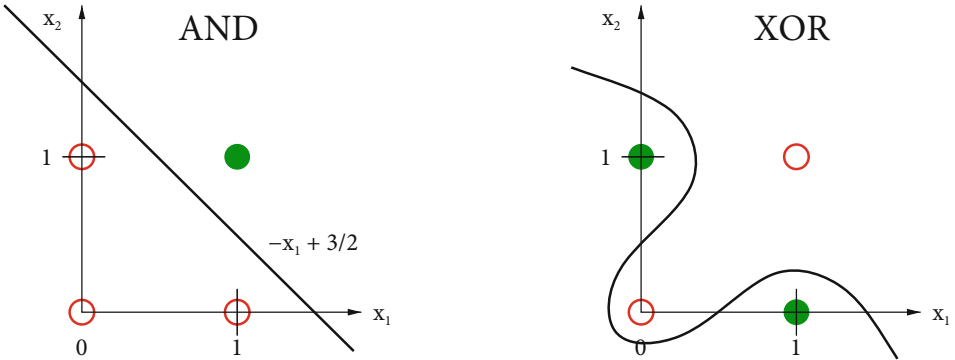
Abb. 8.8 Die boolesche Funktion AND ist linear separabel, XOR hingegen nicht (• \hat{=} wahr, o \hat{=} falsch)
