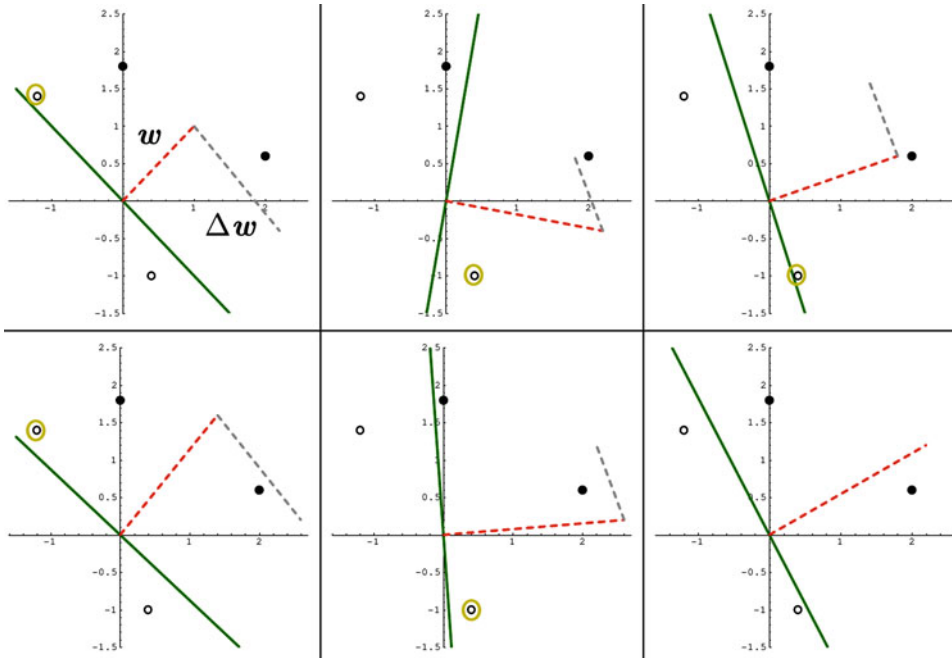
Abb. 8.10 Anwendung der Perzeptronlernregel auf zwei positive (●) und zwei negative (○) Datenpunkte. Die durchgezogene Linie stellt die aktuelle Trenngerade w \cdot x = 0 dar. Die senkrecht darauf stehende gestrichelte Linie ist der Gewichtsvektor w und die zweite gestrichelte Linie der zu w zu addierende Änderungsvektor \Delta w = x oder \Delta w = -x , der sich aus dem jeweils gelb umrandeten Datenpunkt berechnet
