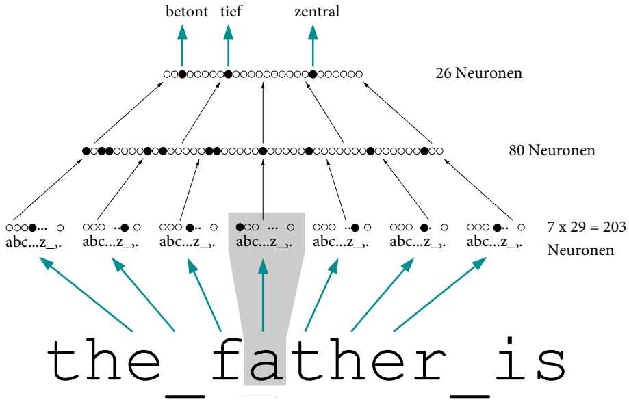
Abb. 9.21 Das NETtalk-Netzwerk bildet einen Text auf seine Ausspracheattribute ab
