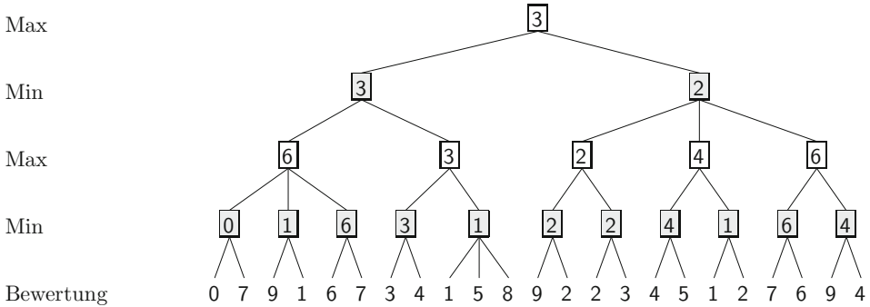
Abb. 6.19 Ein Minimax-Spielbaum mit Vorausschau von 4 Halbzügen
