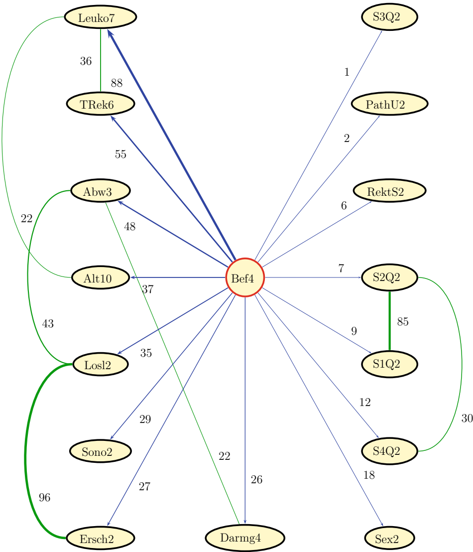
Abb. 7.8 Der aus der Datenbank berechnete Abhängigkeitsgraph
