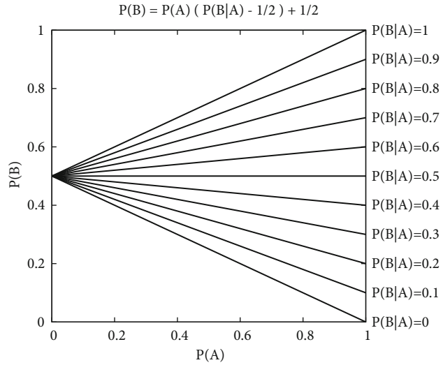
Abb. 7.3 Die Kurvenschar für P(B) in Abhängigkeit von P(A) für verschiedene Werte von P(B|A)
