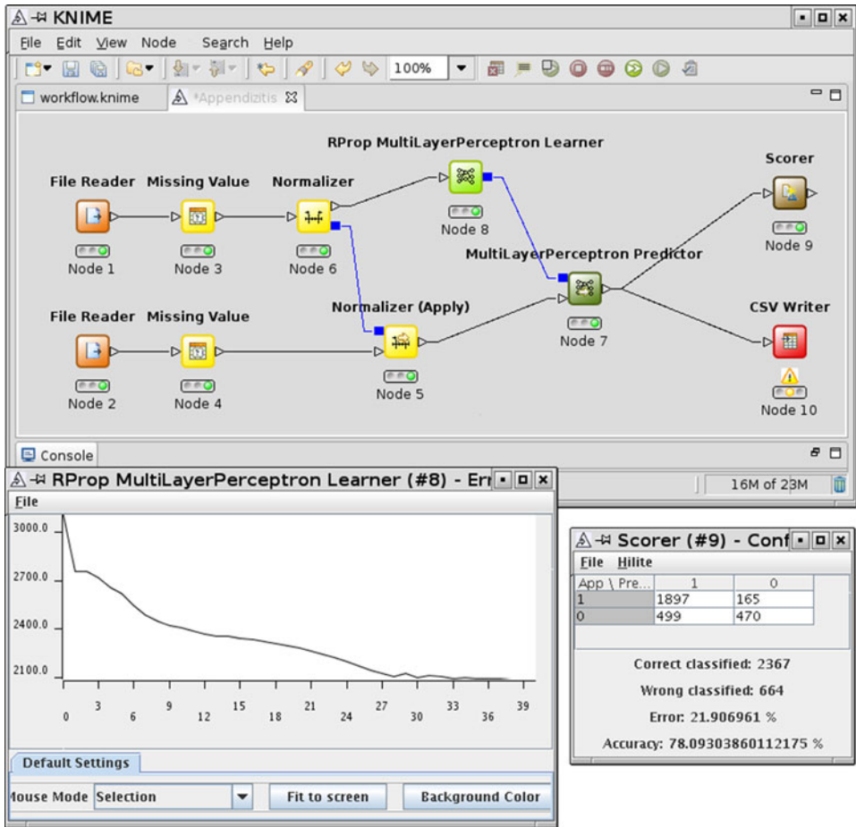
Abb. 8.39 Die KNIME-Benutzeroberfläche mit dem Workflow-Fenster, der Lernkurve und der Konfusionsmatrix
