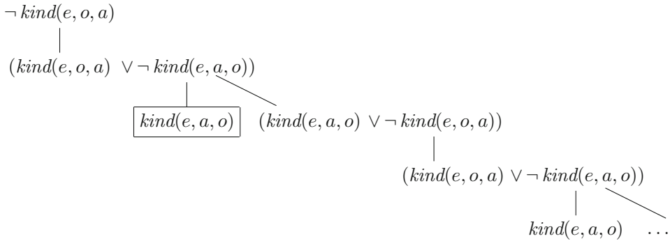
Abb. 5.2 Prolog-Suchbaum für kind(eva, otto, anna)
