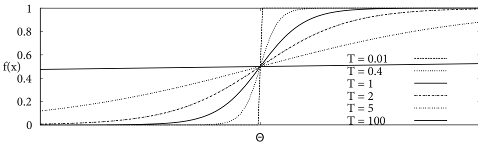
Abb. 9.4 Die Sigmoidfunktion für verschiedene Werte des Parameters T . Man erkennt gut, dass sich im Grenzfall T \rightarrow 0 die Stufenfunktion ergibt
