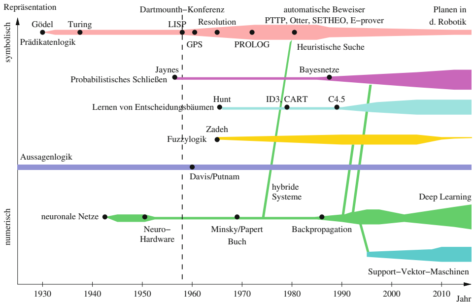
Abb. 1.3 Die Geschichte der verschiedenen KI-Ausrichtungen. Die Breite der Balken soll die Verbreitung der Methode in Anwendungen andeuten
