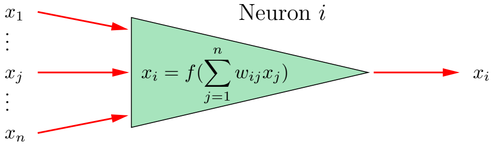
Abb. 9.2 Die Struktur eines formalen Neurons, das auf die gewichtete Summe aller Eingaben die Aktivierungsfunktion f anwendet
