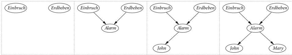
Abb. 7.15 Schrittweiser Aufbau des Alarm-Netzes unter Beachtung der Kausalität
