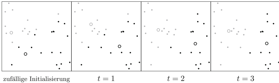
Abb. 8.33 k -Means mit zwei Klassen ( k = 2 ) angewendet auf 30 Datenpunkte. Ganz links die Datenmenge mit den initialen Zentren und nach rechts die Cluster nach jeder Iteration. Nach drei Iterationen ist die Konvergenz erreicht
