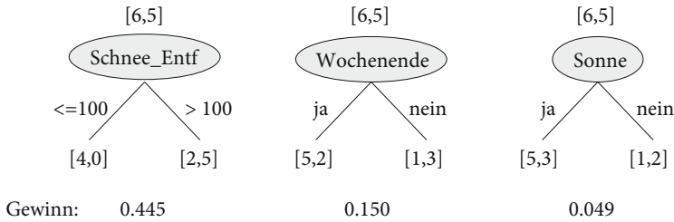
Abb. 8.24 Der für die verschiedenen Attribute berechnete Gewinn spiegelt wider, ob die Aufteilung der Daten durch das jeweilige Attribut zu einer besseren Klassentrennung führt. Je deutlicher die durch die Attribute erzeugten Verteilungen der Daten von der Gleichverteilung abweichen, desto höher ist der Informationsgewinn
