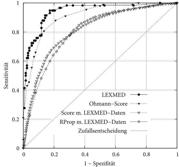
Abb. 7.10 ROC-Kurve von LEXMED verglichen mit dem Ohmann-Score und zwei weiteren Modellen
