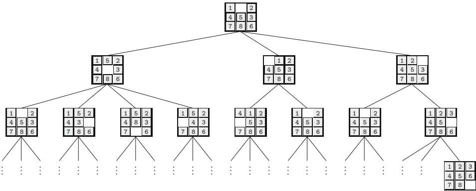
Abb. 6.3 Suchbaum beim 8-Puzzle. Rechts unten ist ein Zielzustand in Tiefe 3 dargestellt. Aus Platzgründen wurden die anderen Knoten auf dieser Ebene weggelassen
