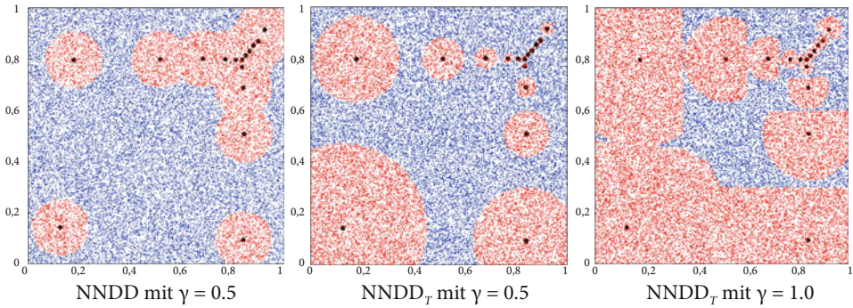
Abb. 8.31 Auf eine Menge von 16 ausgewählten zweidimensionalen Datenpunkten ( schwarze Punkte ) wurde NNDD und \text{NNDD}_T angewendet. Für jeweils 10.000 zufällig gewählte Punkte wurde deren Klassenzugehörigkeit bestimmt. Die rot markierten Punkte wurden als positiv klassifiziert, d. h. der Klasse der Trainingsdaten zugeordnet, die blau markierten dagegen als negativ
