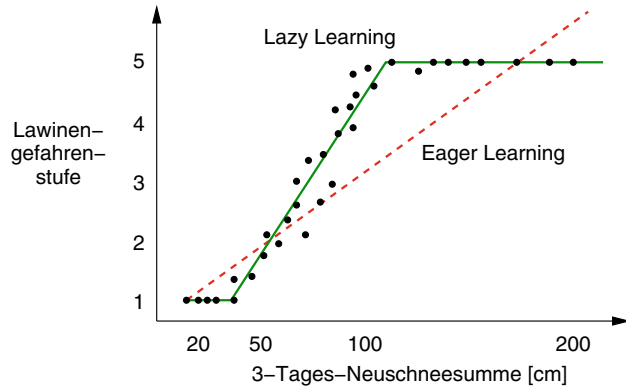
Abb. 8.20 Zur Bestimmung der Lawinengefahr wird aus Trainingsdaten eine Funktion approximiert. Hier im Vergleich ein lokales Modell ( durchgezogene Linie ) und ein globales ( gestrichelt )
