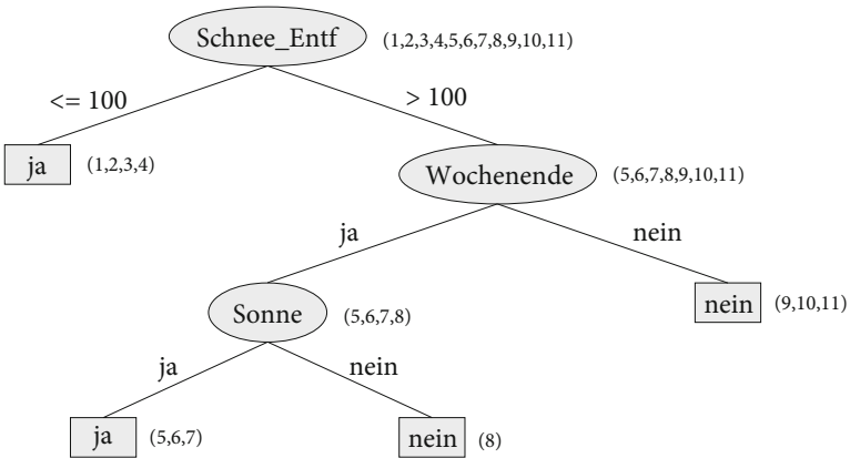
Abb. 8.22 Entscheidungsbaum für das Klassifikationsproblem Skifahren. In den Listen rechts neben den Knoten sind die Nummern der zugehörigen Trainingsdaten angegeben. Man beachte, dass der Blattknoten Sonne = ja nur zwei der drei Beispiele korrekt klassifiziert
