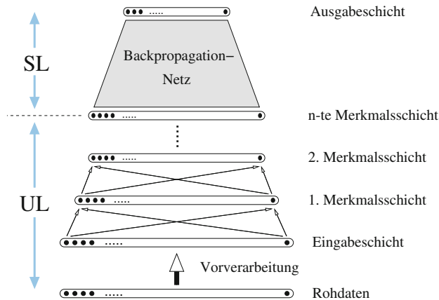
Abb. 9.26 Vereinfachte Architektur eines Deep Learning Netzwerks. Es besteht aus Vorverarbeitung, mehreren Schichten (hier zwei) zur Merkmalsdetektion ohne Lehrer und dann ein klassisches neuronales Netz, das zum Beispiel mit Backpropagation trainiert wird
