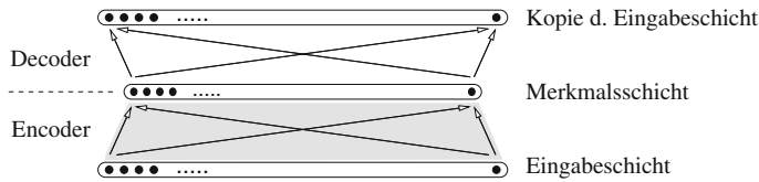
Abb. 9.27 Autoencoder zum Lernen der Gewichte für eine Merkmalsschicht. Ein klassisches Backpropagation-Netz kann hier verwendet werden, um die identische Abbildung der aktuellen Eingabeschicht auf sich selbst zu lernen. Die Merkmale bilden sich beim Lernen in der verdeckten Lage
