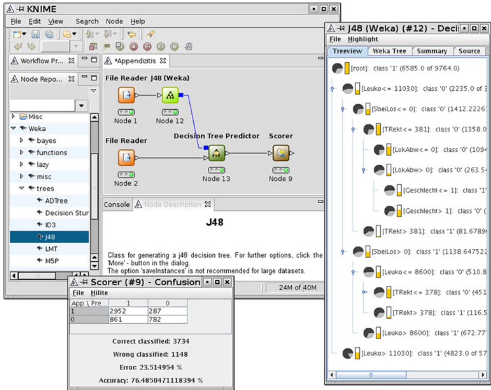
Abb. 8.38 Die KNIME-Benutzeroberfläche mit zwei zusätzlichen Views, die den Entscheidungsbaum und die Konfusionsmatrix darstellen
