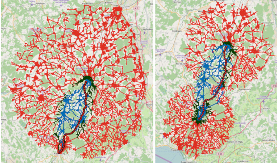
Abb. 6.18 Suchbäume von A* ohne Heuristik (rot), mit Luftlinienabstand (dunkelgrün) und mit Landmarkenheuristik (blau). Das linke Bild zeigt die unidirektionale und das rechte die bidirektionale Suche. Man beachte, dass grüne Kanten von blauen verdeckt werden und rote von grünen und blauen
