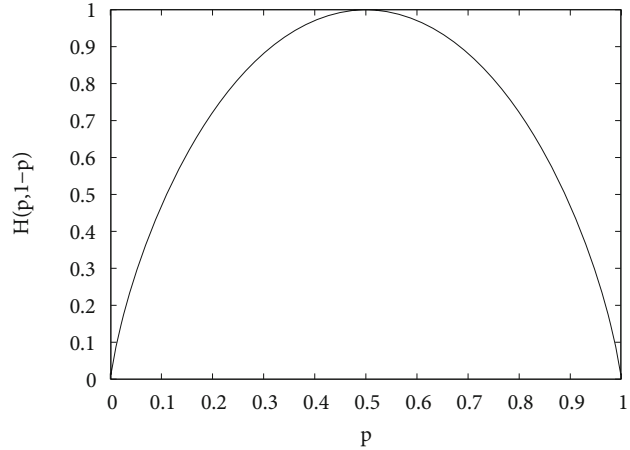
Abb. 8.23 Die Entropiefunktion für den Zweiklassenfall. Man erkennt das Maximum bei p = 1/2 und die Symmetrie bezüglich Vertauschung von p und 1 - p
