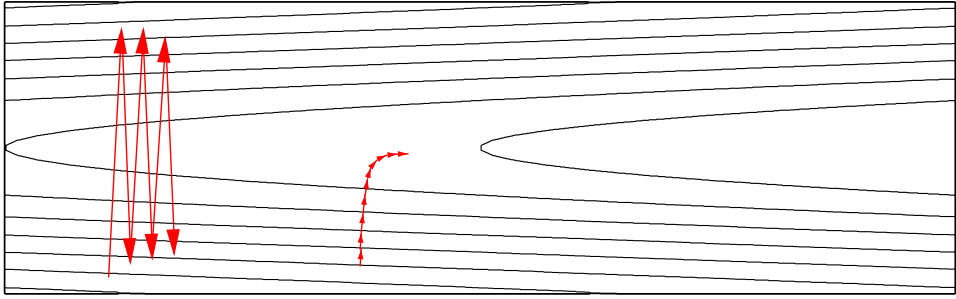
Abb. 9.15 Gradientenabstieg mit großem \eta (links) und sehr kleinem \eta (rechts) in einem nach rechts flach abfallenden Tal. Bei zu großem \eta ergeben sich Oszillationen um das Tal. Bei zu kleinem \eta hingegen wird die Konvergenz in dem flachen Tal sehr langsam
