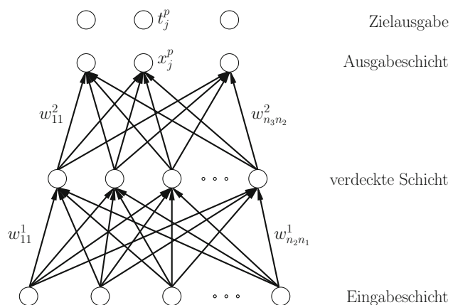
Abb. 9.18 Ein dreilagiges Backpropagation-Netz mit n_1 Neuronen in der ersten, n_2 Neuronen in der zweiten und n_3 Neuronen in der dritten Schicht
