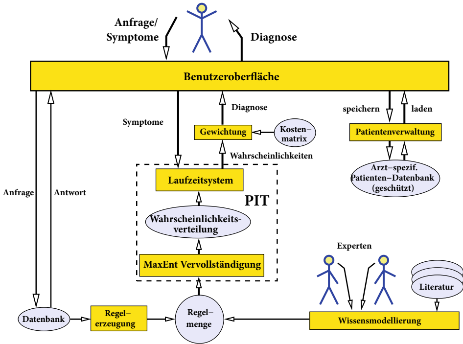
Abb. 7.7 Aus der Datenbank sowie aus Expertenwissen werden Regeln generiert. MaxEnt erzeugt daraus eine vollständige Wahrscheinlichkeitsverteilung. Auf eine Anfrage des Benutzers wird für jede mögliche Diagnose eine Wahrscheinlichkeit berechnet. Mit Hilfe der Kostenmatrix (siehe Abschn. 7.3.5) wird dann eine Entscheidung vorgeschlagen
