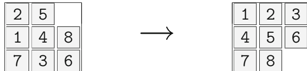
Abb. 6.2 Mögliche Start- und Zielzustände des 8-Puzzle
