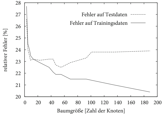
Abb. 8.26 Lernkurve von C4.5 auf den Appendizitisdaten. Man erkennt deutlich die Überanpassung bei Bäumen mit mehr als 55 Knoten
