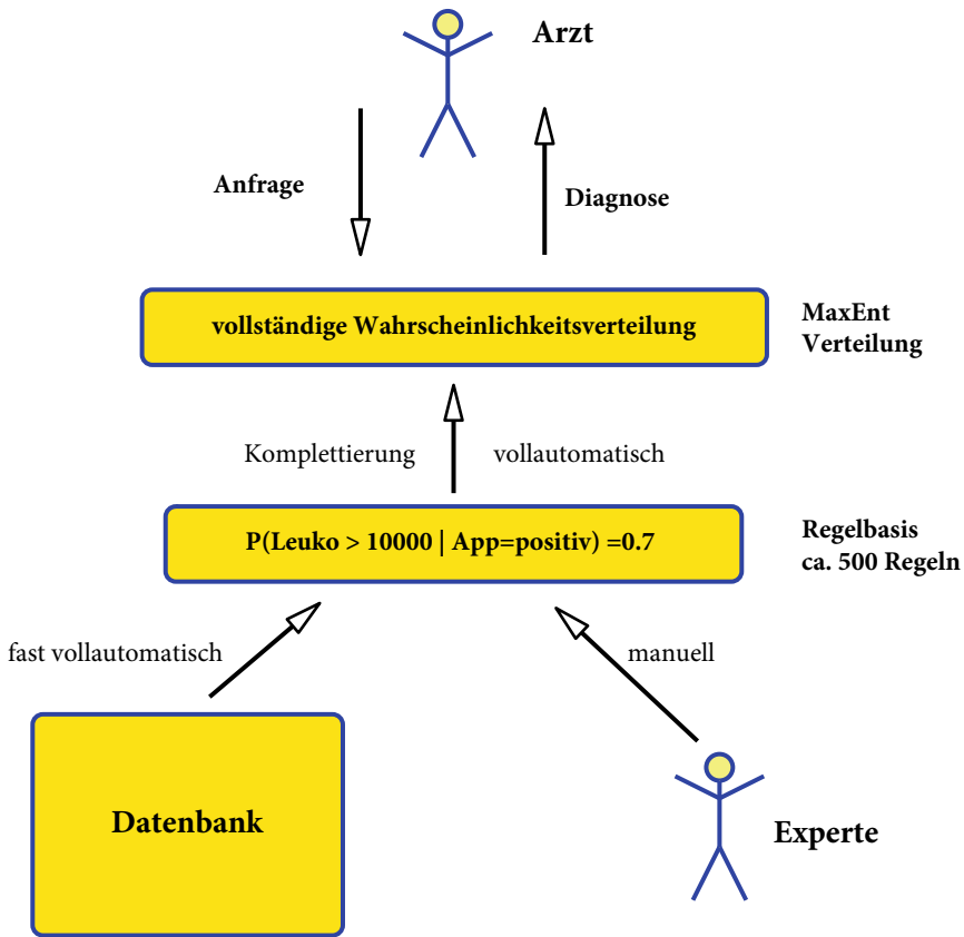
Abb. 7.5 Aus Daten und Expertenwissen werden Wahrscheinlichkeitsregeln generiert, die in einer Regelbasis (Wissensbasis) integriert und anschließend mit der MaxEnt-Methode vervollständigt werden
