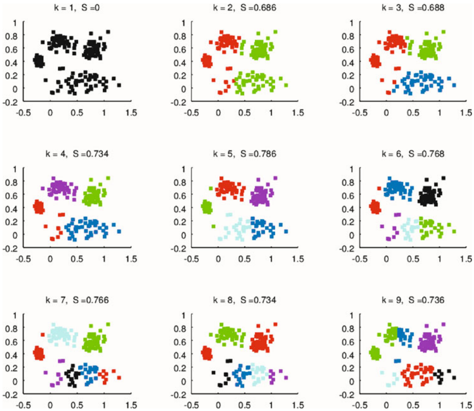
Abb. 8.36 Ergebnisse des OMRk-Algorithmus für k = 2 bis 9. Der beste Wert mit S = 0,786 wurde gefunden für k = 5
