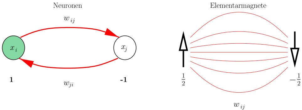
Abb. 9.8 Vergleich zwischen der neuronalen und der physikalischen Interpretation des Hopfield-Modells
