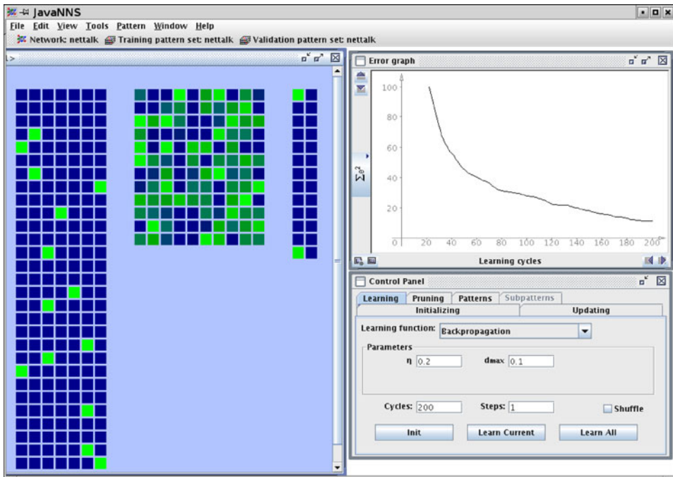
Abb. 9.22 Das NETtalk-Netzwerk in JNNS. Im linken Fenster von links nach rechts erkennt man die 7 · 29 Eingabeneuronen, 80 verdeckte und 26 Ausgabeneuronen. Aufgrund der großen Zahl sind die Gewichte im Netz ausgeblendet. Rechts oben ist eine Lernkurve mit der zeitlichen Entwicklung des quadratischen Fehlers zu sehen
