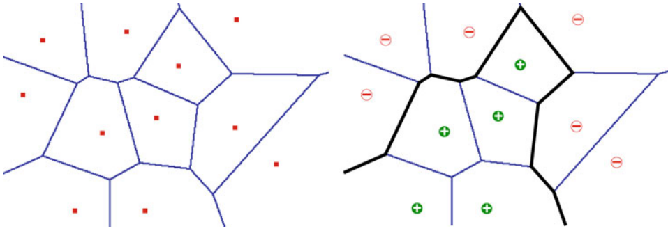
Abb. 8.14 Eine Punktmenge zusammen mit ihrem Voronoi-Diagramm ( links ) und die daraus erzeugte Linie zur Trennung der beiden Klassen M_+ und M_- .
