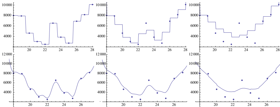
Abb. 8.19 Vergleich der k -Nearest-Neighbour-Methode ( obere Reihe ) mit k = 1 ( links ), k = 2 ( Mitte ) und k = 6 ( rechts ), mit der abstandsgewichteten Variante ( untere Reihe ) mit \alpha = 20 ( links ), \alpha = 4 ( Mitte ) und \alpha = 1 ( rechts ) auf einer eindimensionalen Datenmenge
