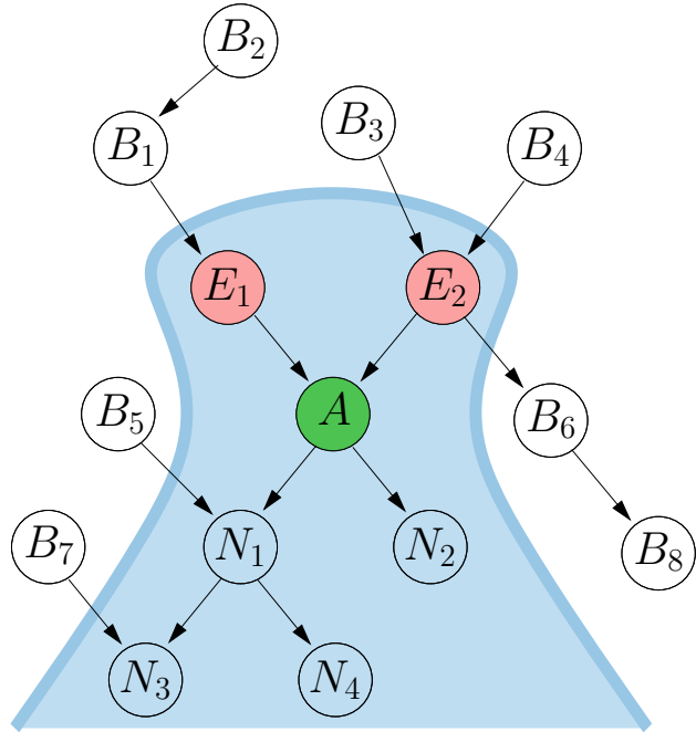
Abb. 7.17 Beispiel für die bedingte Unabhängigkeit in einem Bayes-Netz. Sind die Elternknoten E_1 und E_2 gegeben, so sind alle Nichtnachfolger B_1, \dots, B_8 unabhängig von A
