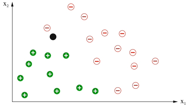
Abb. 8.13 In diesem Beispiel mit negativen und positiven Trainingsbeispielen weist die Nearest Neighbour-Methode dem neuen schwarz markierten Punkt die negative Klasse zu
