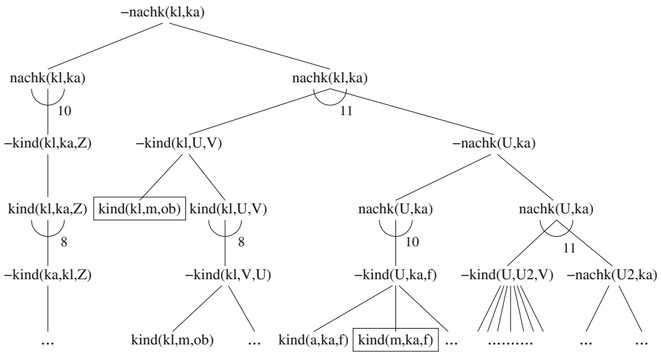
Abb. 5.3 Und-Oder-Baum für nachk(klaus, katrin)
