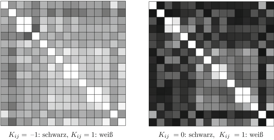
Abb. 8.6 Die Korrelationsmatrix als Dichteplot. Im linken Diagramm steht dunkel für negativ und hell für positiv. Im rechten Bild wurden die Absolutbeträge eingetragen. Hier bedeutet schwarz K_{ij} \approx 0 (unkorreliert) und weiß |K_{ij}| \approx 1 (starke Korrelation)
