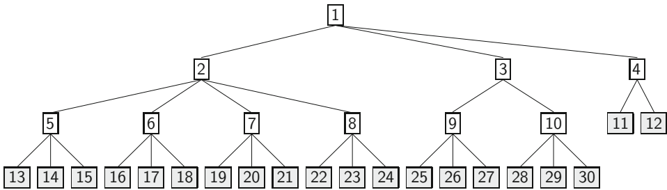
Abb. 6.7 Breitensuche während der Expansion der Knoten der dritten Ebene. Die Knoten sind nummeriert nach der Reihenfolge ihrer Erzeugung. Die Nachfolger der Knoten 11 und 12 sind noch nicht erzeugt
