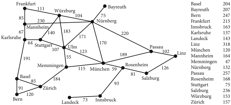
Abb. 6.14 Städtegraph mit Luftlinienentfernungen aller Städte nach Ulm
