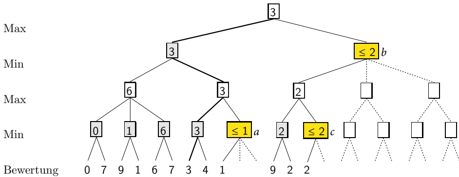
Abb. 6.20 Ein Alphabeta-Spielbaum mit Vorausschau von 4 Halbzügen. Die gestrichelten Teile des Suchbaumes werden nicht traversiert, denn sie haben keinen Einfluss auf das Ergebnis
