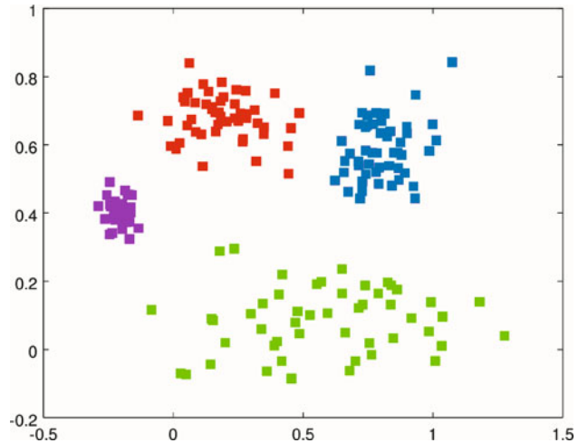
Abb. 8.37 Eine mit dem EM-Algorithmus erzeugte Partition für k = 4
