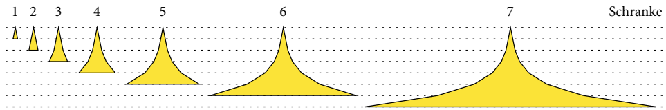
Abb. 6.10 Schematische Darstellung der Entwicklung der Suchbäume bei Iterative Deepening mit Schranken von 1 bis 7. Die Breite der Bäume entspricht einem Verzweigungsfaktor von 2
