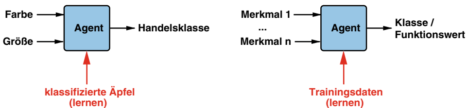
Abb. 8.4 Funktionale Struktur des lernenden Agenten für die Apfelsortierung ( links ) und allgemein ( rechts )
