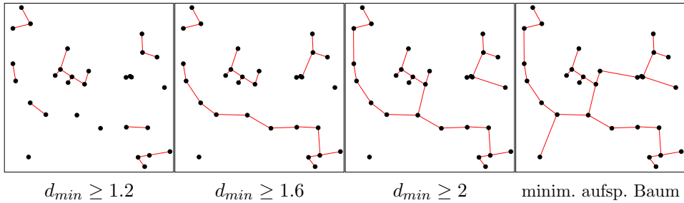
Abb. 8.35 Der Nearest Neighbour-Algorithmus, angewandt auf die Daten aus Abb. 8.33 auf verschiedenen Ebenen mit 12, 6, 3, 1 Clustern
