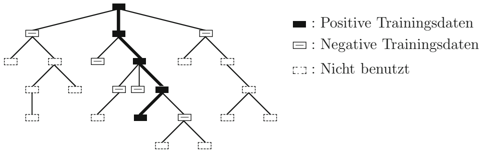
Abb. 9.23 Suchbaum mit einem erfolgreichen Pfad, dessen Knoten positiv bewertet werden und die negativ bewerteten nicht erfolgreichen Abzweigungen
