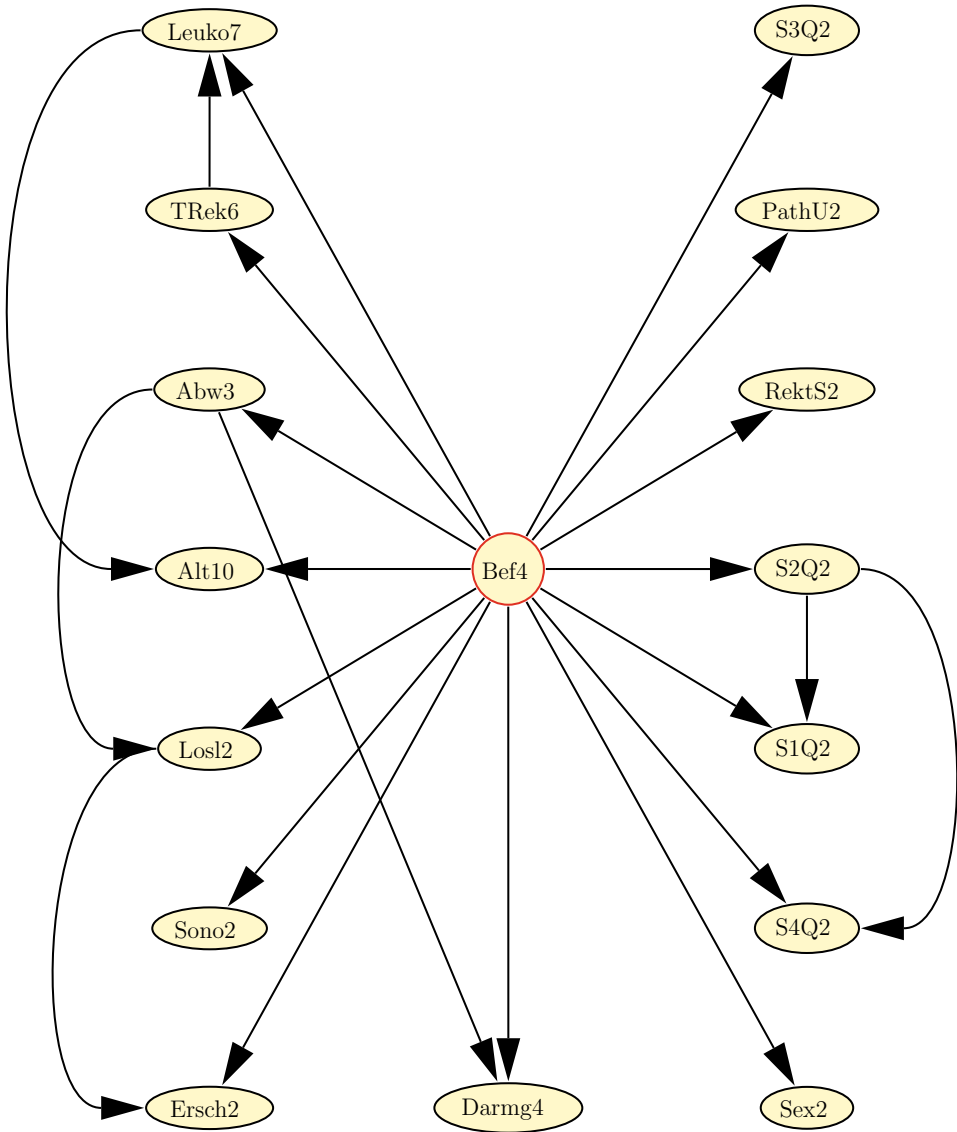
Abb. 7.14 Bayes-Netz für die LEXMED-Anwendung
