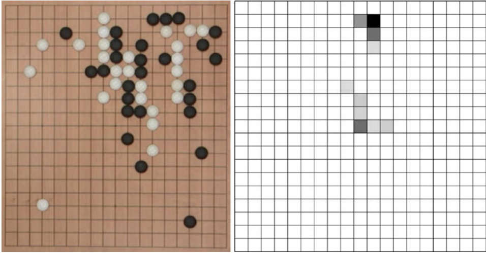
Abb. 10.13 Dichteplot (rechts) der Zugwahrscheinlichkeit p_\sigma(a | s) für den Spieler mit den weißen Steinen in der links gezeigten Stellung. Für alle weißen Felder ist p_\sigma(a | s) = 0 . Je dunkler ein Feld desto höher die Bewertung für einen Zug von Weiß auf dieses Feld
