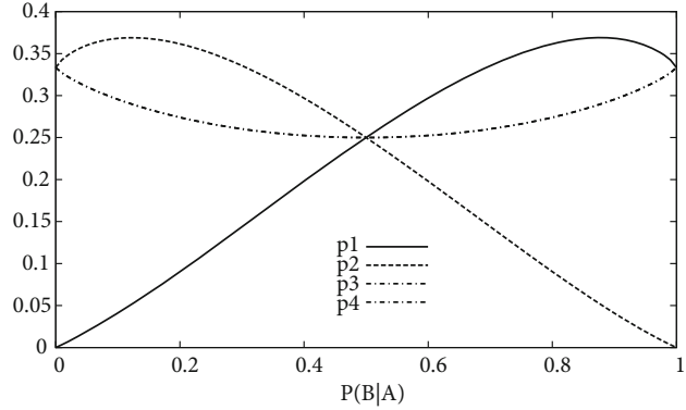
Abb. 7.4 p_1, p_2, p_3, p_4 in Abhängigkeit von \beta
