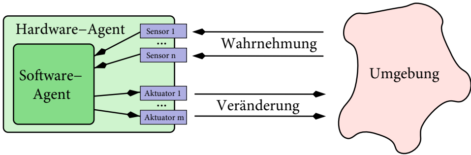
Abb. 1.6 Ein Hardware-Agent
