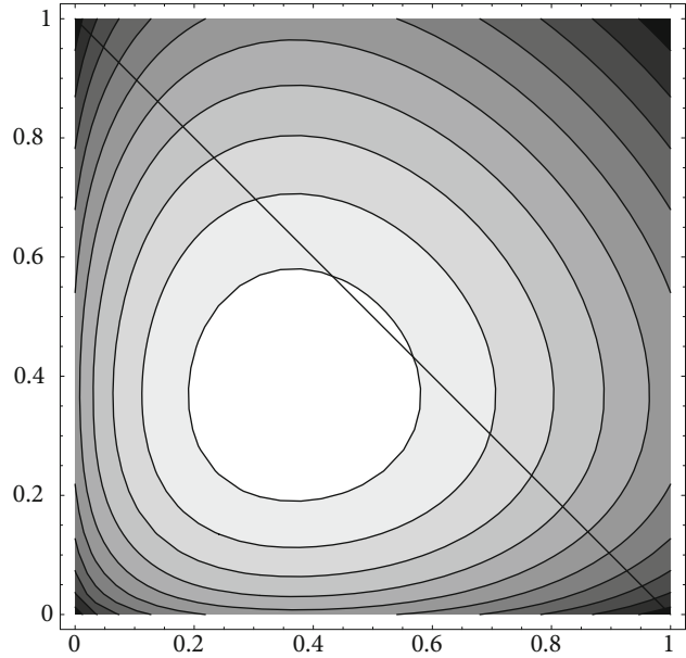
Abb. 7.2 Höhenliniendiagramm der zweidimensionalen Entropiefunktion. Man erkennt, dass sie im gesamten Einheitsquadrat streng konvex ist und dass sie ein isoliertes globales Maximum besitzt. Eingezeichnet ist außerdem die Nebenbedingung p_3 + p_4 = 1 als Spezialfall der hier relevanten Randbedingung p_3 + p_4 - 1 + \alpha = 0 für \alpha = 0
