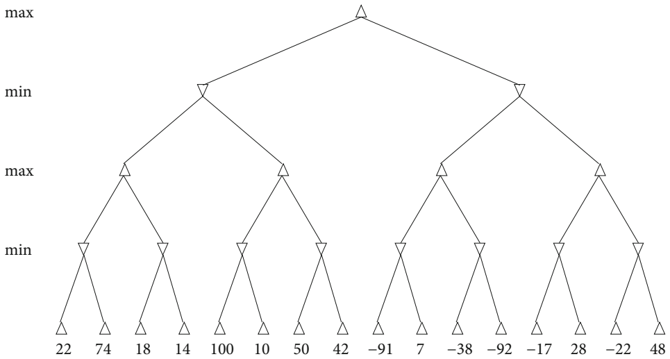
Abb. 6.23 Minimax-Suchbaum
