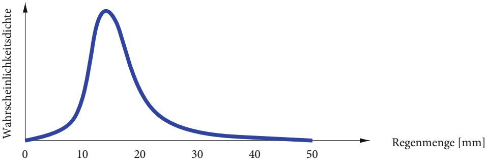
Abb. 4.3 Wahrscheinlichkeitsdichte der stetigen Variable Regenmenge
