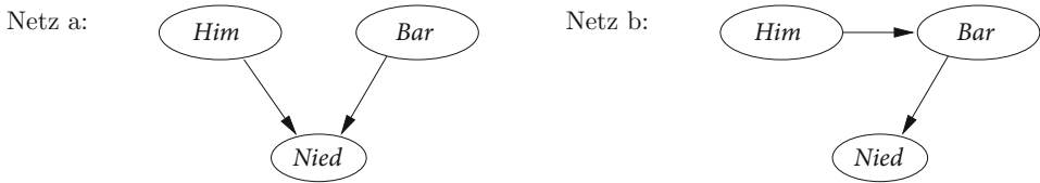
Abb. 8.28 Zwei Bayes-Netze zur Modellierung des Wettervorhersage-Beispiels aus Aufgabe 7.3
