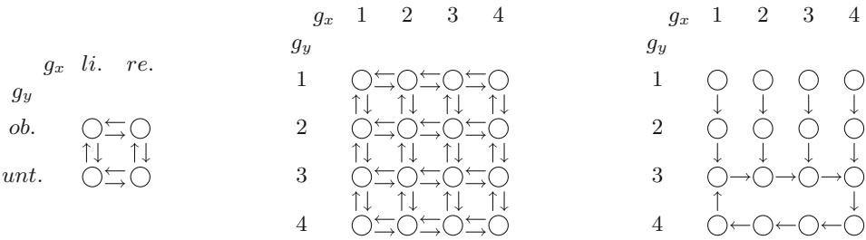
Abb. 10.3 Der Zustandsraum des Beispielroboters im Fall von je zwei möglichen Positionen der Gelenke ( links ) und im Fall von je vier horizontalen und vertikalen Positionen ( Mitte ). Im rechten Bild ist eine optimale Strategie angegeben
